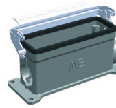
Base Larga de 1 Gancho Con 2 Entradas 29372-2305S
